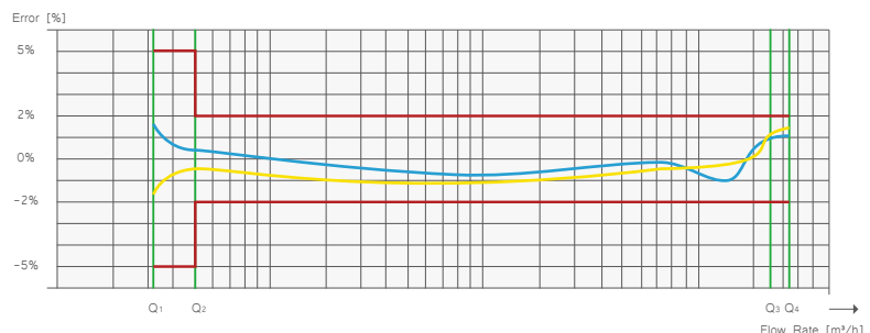
BECO Y Curva de precisión del medidor de agua ultrasónico
